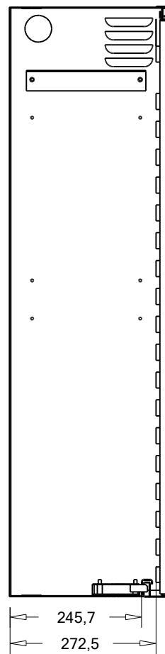
Przekrój J-J
