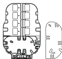
Kaseta przełączeniowa C6 4 adaptory duplex SC lub 2 adaptory quad (poczwórne) LC
